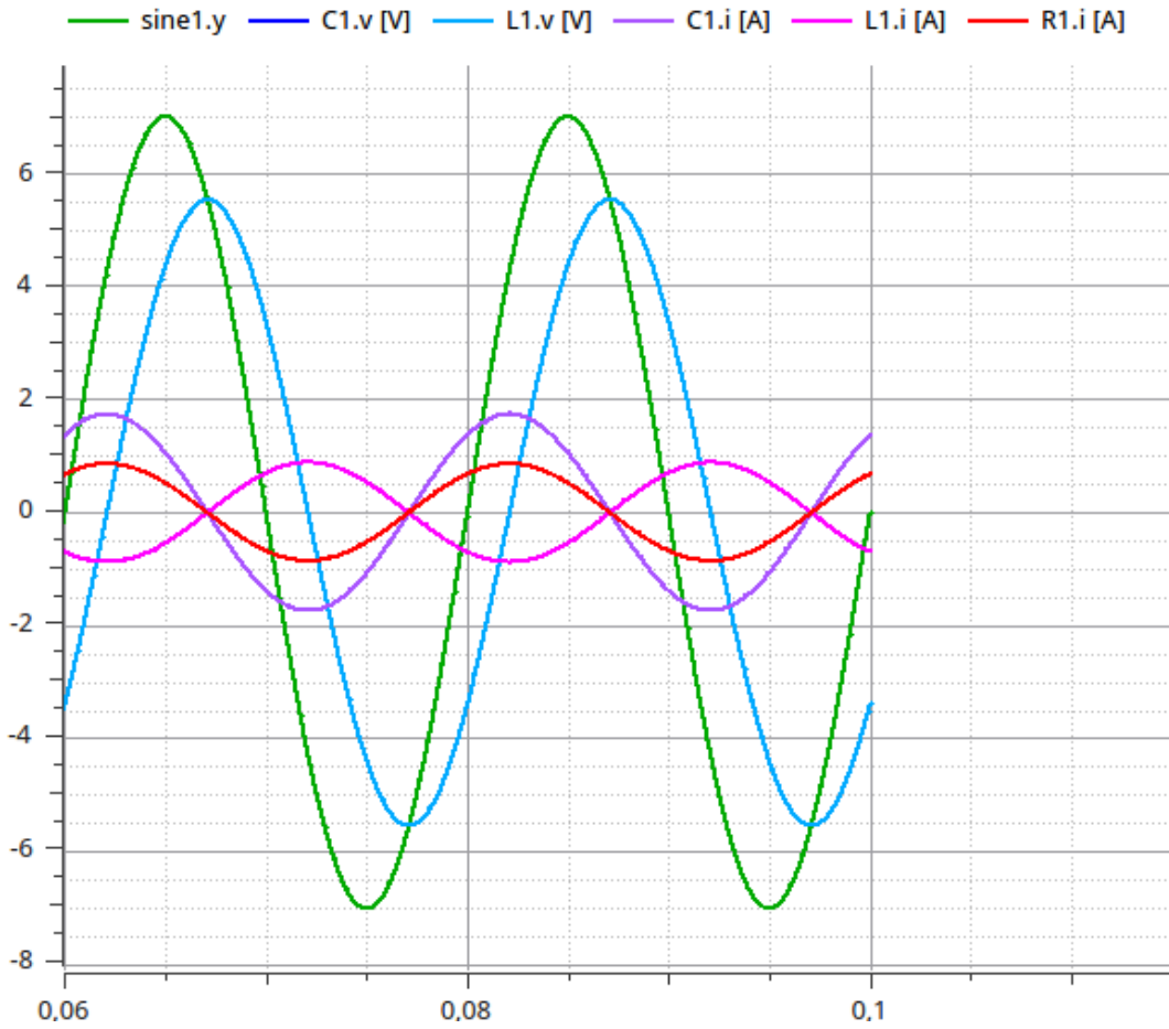
Oscillogramme de l'application « lois des mailles et des noeuds »
