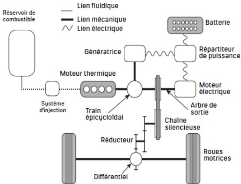
Schéma simplifié du système technique
